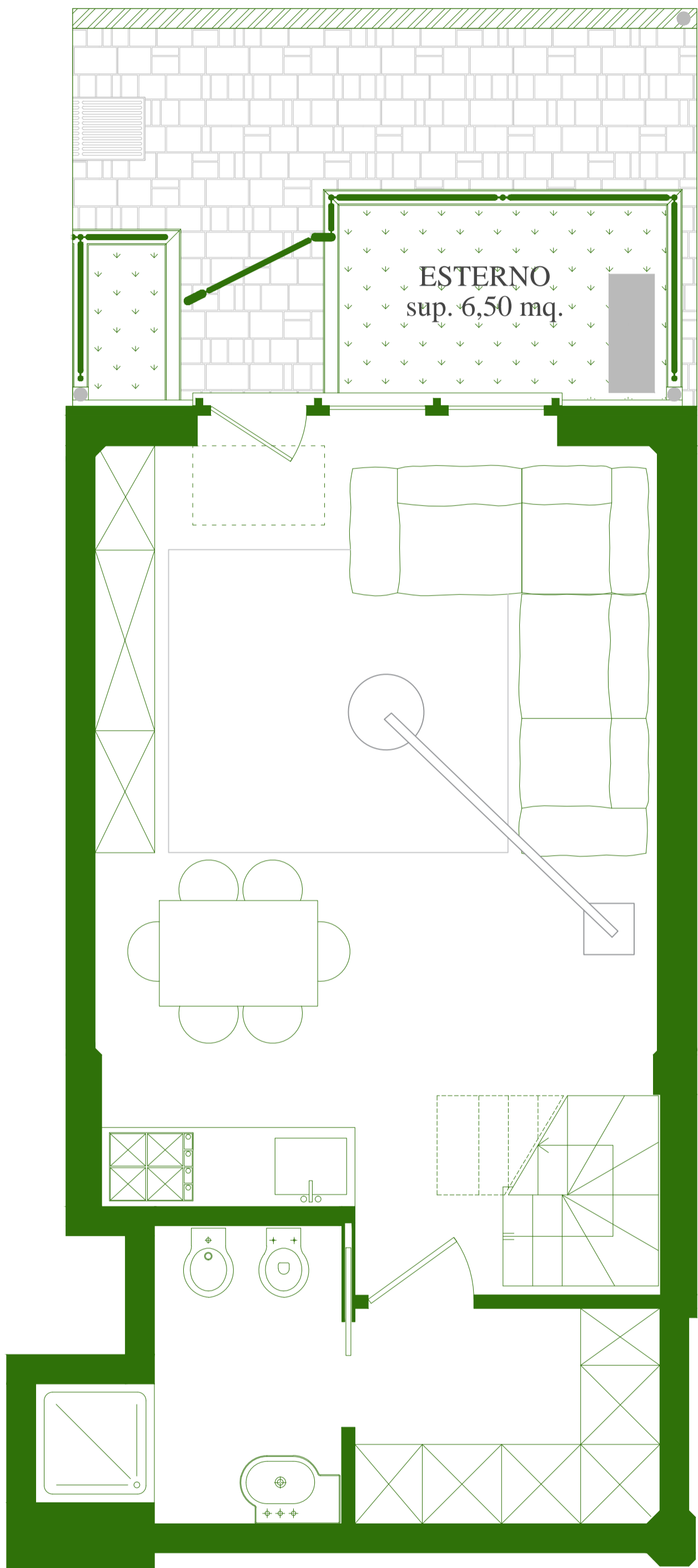
14 APPARTAMENTO tipo G
